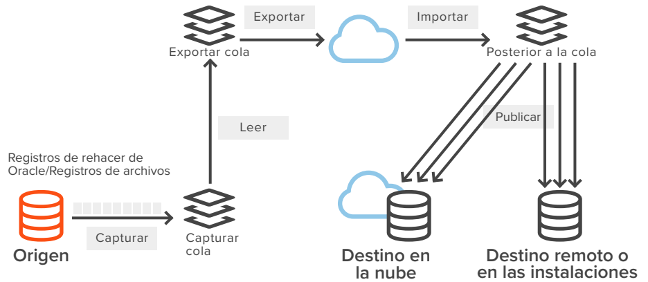
El proceso de replicación de datos de SharePlex
